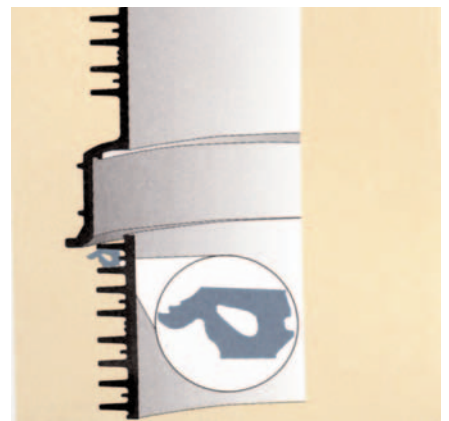
3. Dichtelement DN 1000 in die Kammer zwischen 1. und 2. Rippe (siehe Bild) an der Oberseite gleichmäßig einlegen. Dichtelement auf Beschädigungen und richtigen Sitz überprüfen.
