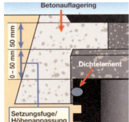
9. Dichtelement DN 625 in oberstes Rippental am Konus einlegen. Schrift nach oben. Betonauflagering DN 625 am Schachtkonus aufsetzen und Abdeckung oder Ausgleichsringe auflegen.
