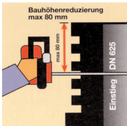
8. Zur Bauhöhenreduzierung kann der Schachtkonus am Einstieg um max. 80 mm gekürzt werden. Schachtröhre können in 125 mm Schritten an markierten Stellen gekürzt werden.
