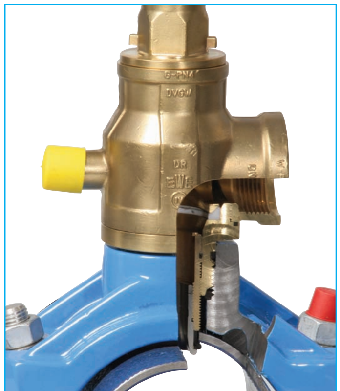
Kugel-Ventil-Anbohrarmatur für AZ-, Guss- und Stahlrohr mit Bohrloch-Dichthülse im Schnitt
