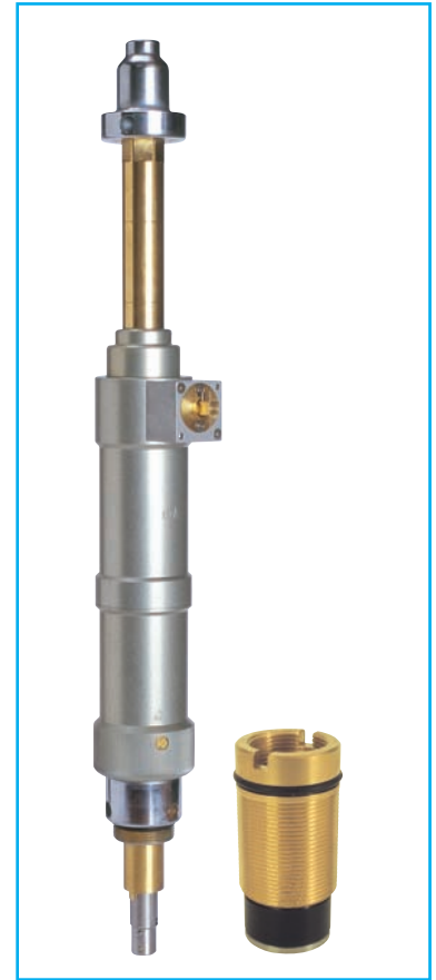
Bohrloch-Dichthülsen-Setzgerät mit Bohrloch-Dichthülse
